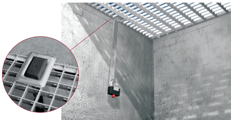
^ Stabile Abhebsicherung
