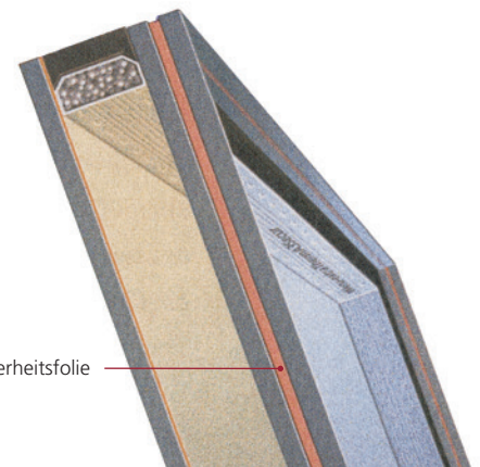
^ Angrifffhemmendes Verbundsicherheitsglas
